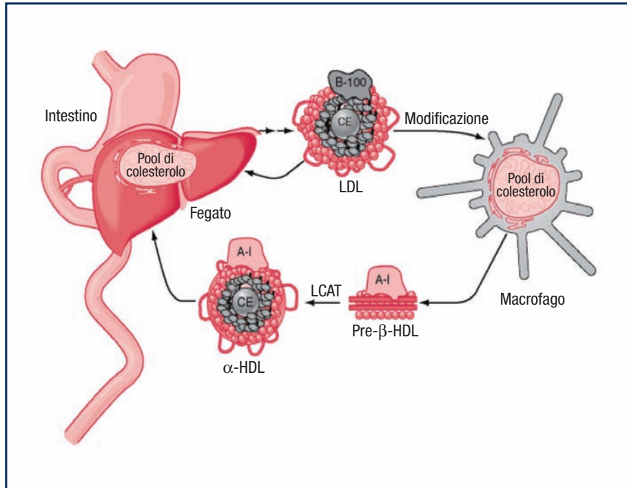
FIGURA 5 LDL e trasporto inverso del colesterolo
