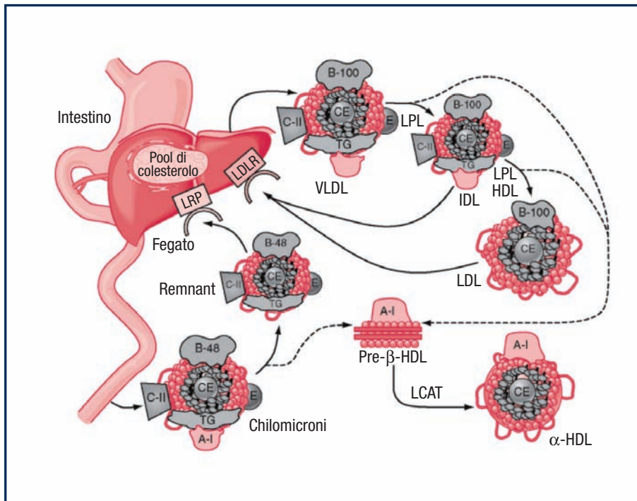
FIGURA 4 Relazione tra lipoproteine ricche di trigliceridi ed HDL
