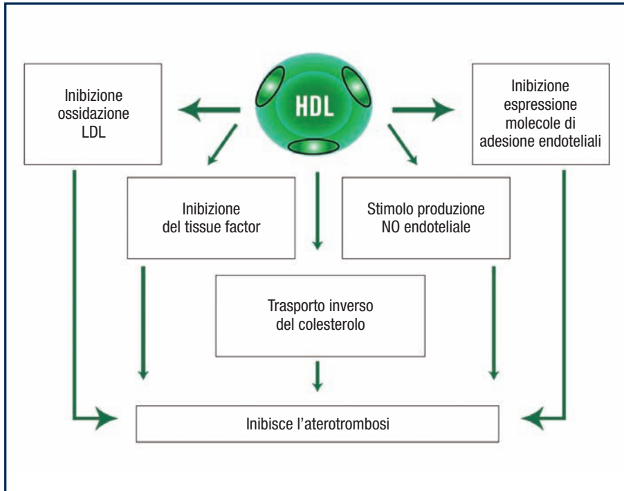
FIGURA 3 Effetti protettivi delle HDL
