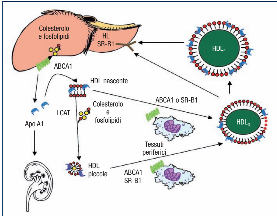
FIGURA 1 Ciclo metabolico delle HDL
