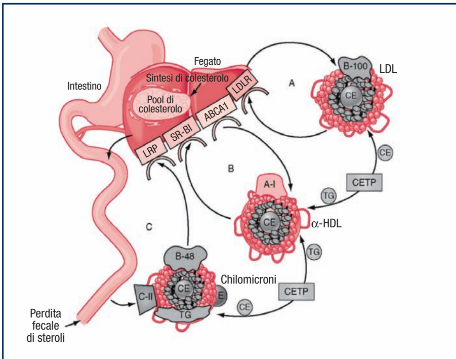
FIGURA 8 Tre cicli integrati controllano il pool epatico di colesterolo
