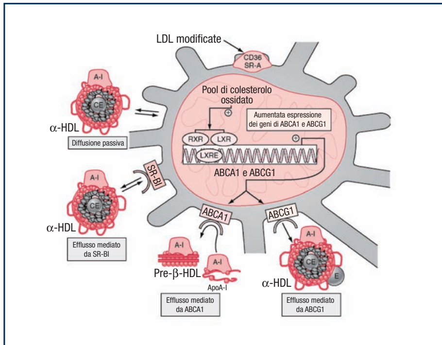
FIGURA 6 Vie di efflusso del colesterolo da macrofagi
