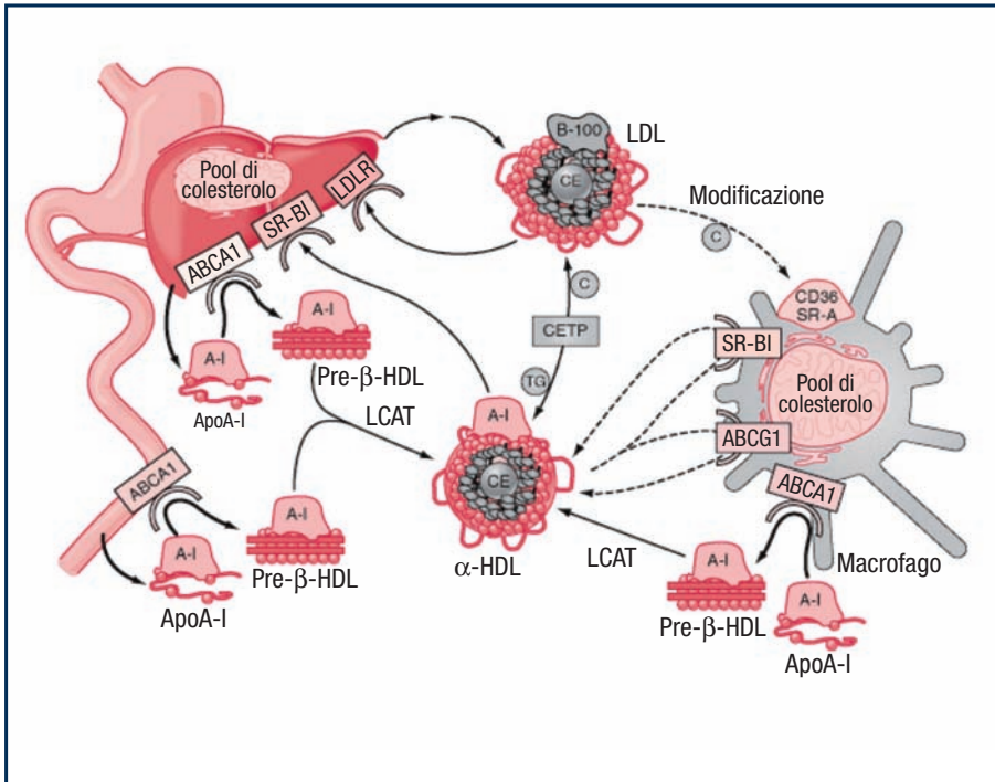
FIGURA 7 I livelli di colesterolo intracellulari di fegato e macrofagi sono modulati dalle HDL
