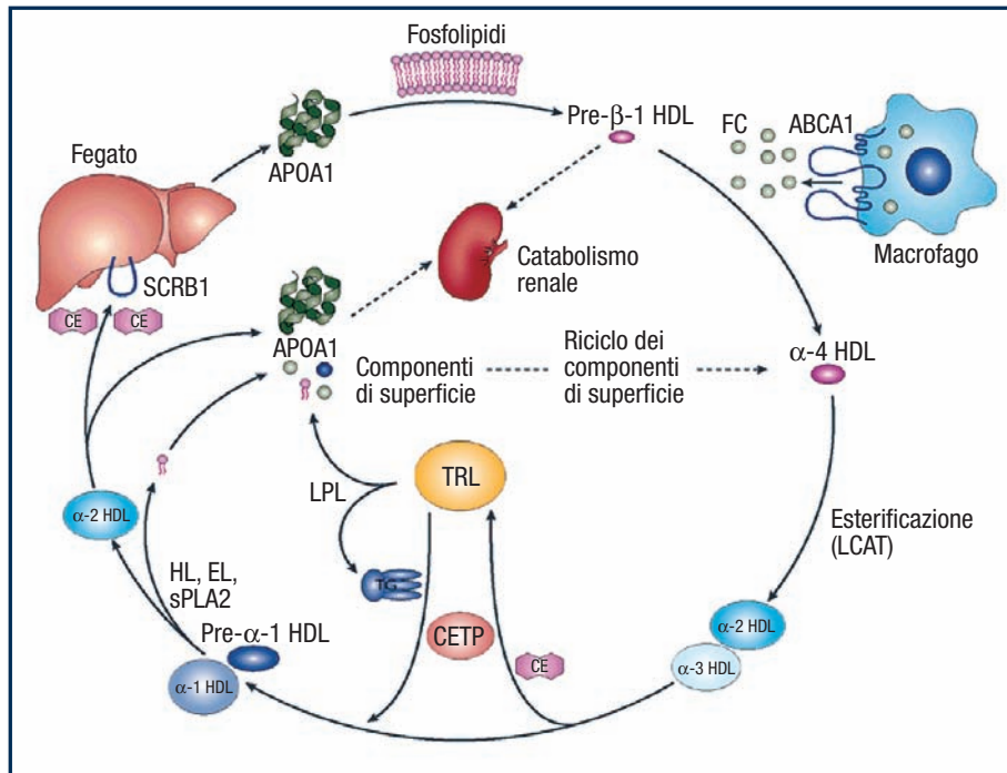
FIGURA 2 Trasporto inverso del colesterolo (RCT)
